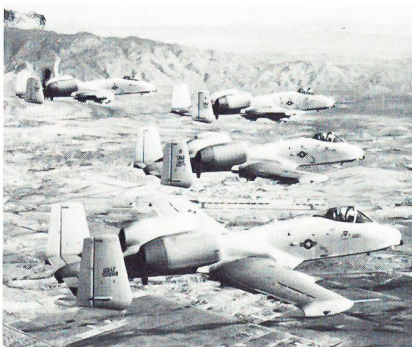
Mit dem Luftnahunterstützungsflugzeug A-10 bekämpften die amerikanischen Luftstreitkräfte Panzeransammlungen, SCUD-Stellungen, Fahrzeugkolonnen, Bunker usw. Zum Einsatz gelangten unter anderen die Familie von Luft/Boden-Lenk Waffen AGM-65 Maverick und vor allem die integrierte 30-mm-Gatling-Maschinenkanone.
