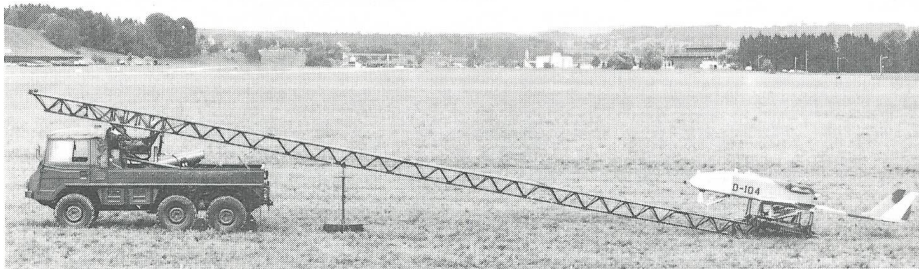
Hydromechanisches Startkatapult, aufgebaut auf Geländefahrzeug Pinzgauer 6x6. Startbereite Drohne am hinteren Ende des Katapultes.
