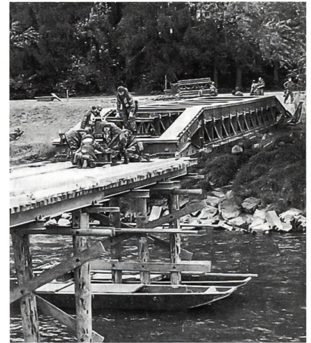
Rückzugsarbeiten an der «Kombi-Brücke» bei Amlikon. Pontons dienen als Arbeitsbühne.
