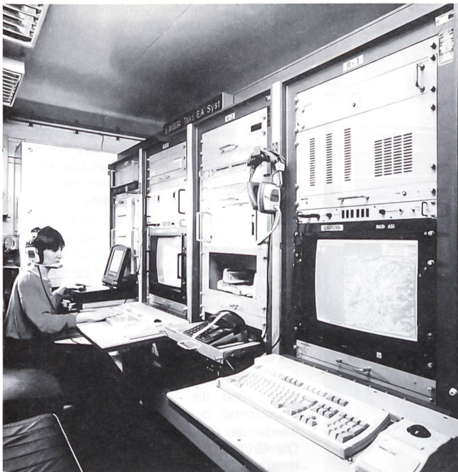
Die Auswertungszentrale, eingebaut im Geländefahrzeug «Duro», dient der Auswertung der «Taktischen Aufklärung».
