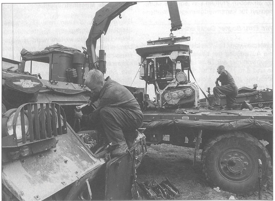
Motorpanne im Feld. Auf dem Bild: Auswechseln eines ganzen Motors im Feld.
