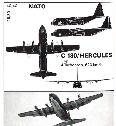
C-130 Hercules
