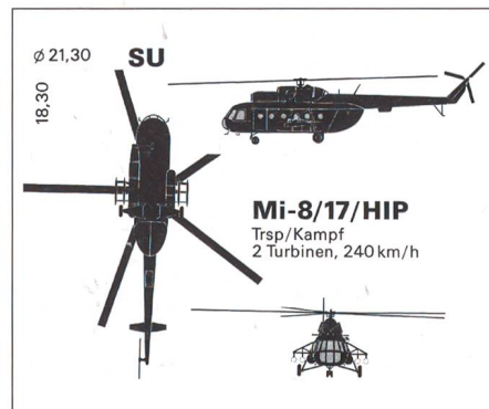
Mi 8/17 Hip
