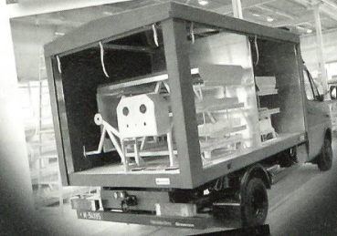
FHS-Spezial-Wechselaufbau
