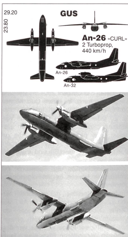
AN-26
