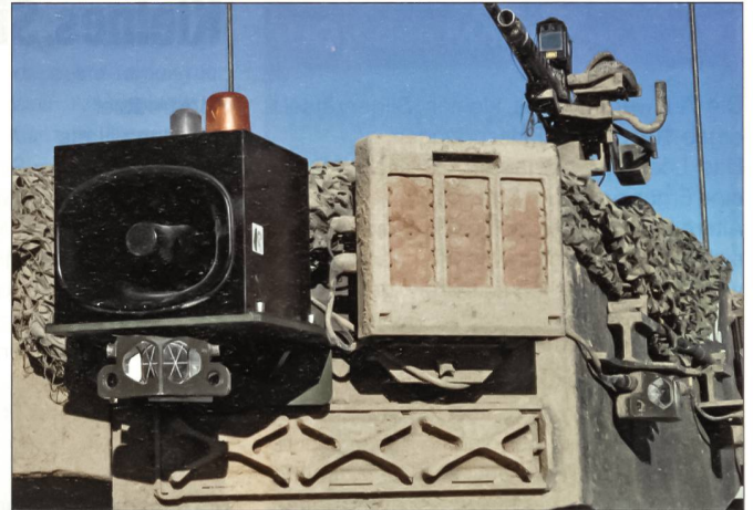
Der neue Laserschusssimulator, installiert am Kampfpanzer 87 Leopard WE.
