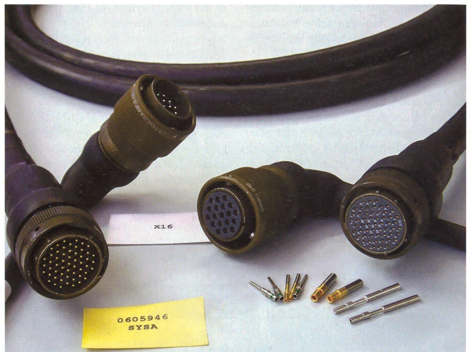
Die Abbildung zeigt, wie anspruchsvoll die Schnittstelle Kabel-Stecker für militärische Zwecke konstruiert ist.
