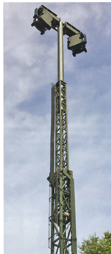
Der Kommunikationspanzer hat den Mast aufgerichtet. Oben Richtstrahlgeräte R-905, gerichtet auf das Relais, von dem die Verbindung über den Knoten ins IMFS (Integriertes Militärisches Fernmeldesystem) führt. IMFS-Standort geheim.
