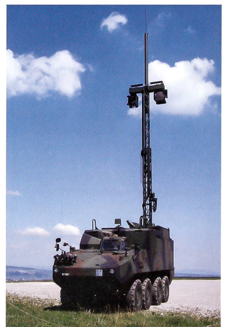
Piranha 3 RAP-Panzer.
