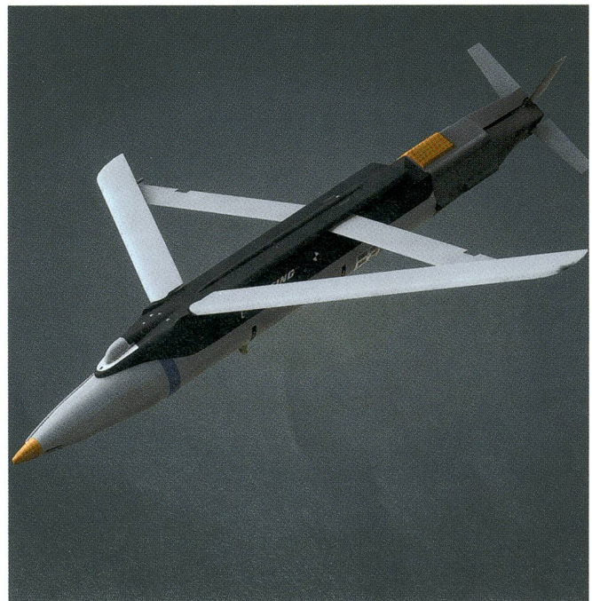
Die amerikanische Durchmesserbombe GBU-39.
