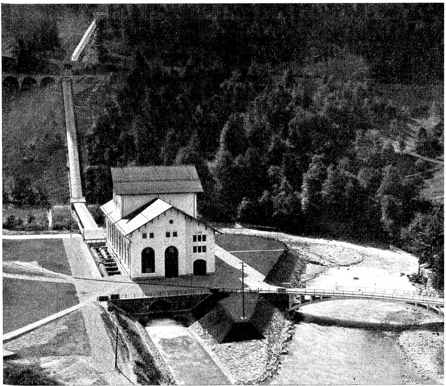
Hochdruckwerk an der Albula , Graubünden, gebaut 1910. Das Wasser stürzt aus großer Höhe zu den Turbinen hinunter und bringt die Schaufelräder in Schwung. Vorn sieht man, wie es unter dem Turbinenhaus wieder hervorkommt und rechts in die Albula mündet.
