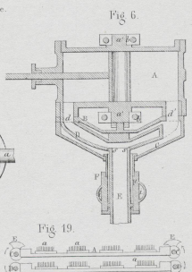
Jefferys oscillirende Maschine.
