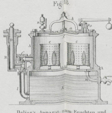
Delize's Apparat zum Feuchten und Trocknen der Woll Kutzer.
