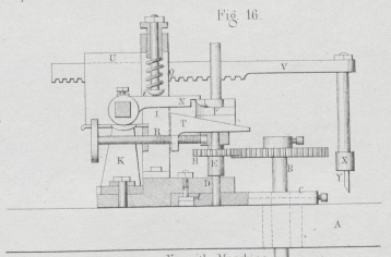
Neomiths Maschine zum Behauen von Mirlsteinen.
