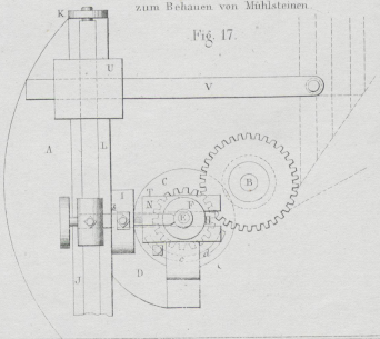
Neomiths Maschine zum Behauen von Mirlsteinen.
