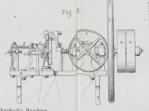
Rauschenbachs Maschine zur Verfertigung der Stecknadeln.
