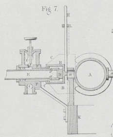
Jefferys oscillirende Maschine.
