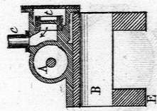
Fig. 6. Schnitt 7-8.
