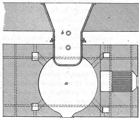
Fig. 3. Grundriss nach A-B der Fig. 2.
