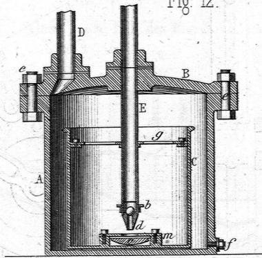
Wasserfang bei Dampfkesseln. Fig. 12.
