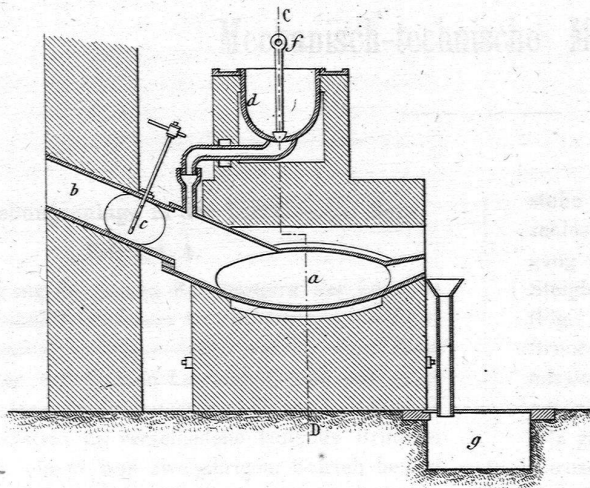
Fig. 2. Schnitt nach C-D der Fig. 1.
