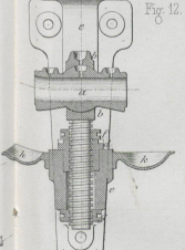
Wandlager Leichte Transmissionswellen
