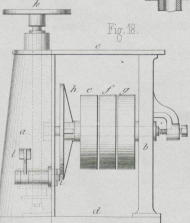
Fischer's Aufu. Abtreibmaschine für Thorwaaren.
