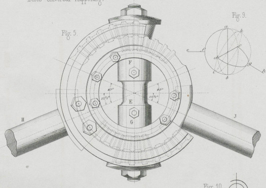
Blees' Universal Kuppelung.
