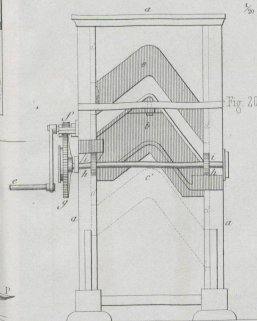
Walkmaschine für Stiefelschäfte.
