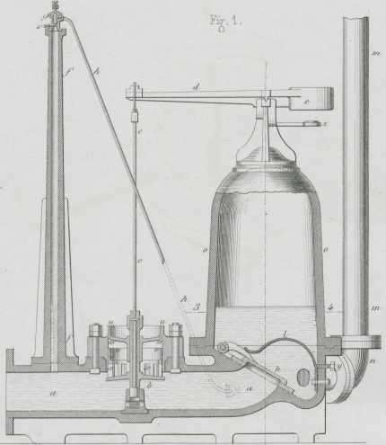
Bollee's Stossheber.
