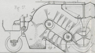
Apparat zum Messen u. Wägen des Getreides.
