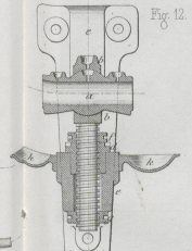
Wandlager
