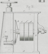
Fischer's Aufu. Abdrehmachine für Thorwaaren.
