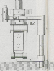
Claudius' Zuggeschwindigkeitmesser.
