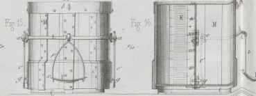
Apparat zum Messen u. Wägen des Getreides.
