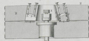
Fig. 13. Lefevre's Muhlsteine mit Quetschwalzen.
