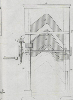
Walkmaschine für Stiefelschäfte.
