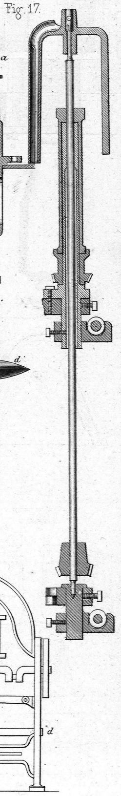
Pfaff's Führungsbüchse
