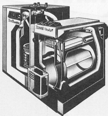
Hoval UnoLyt Niedertemperatur- Öl-/Gaskessel mit Beistellboiler Hoval CombiVal
