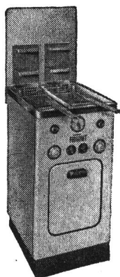
Modell Ze-Rapide Masse: 42×53×80 cm 2 Ölbassins zu je 5 l Inhalt Anschlusswert der 2 getrennten Heizungen je 3,5 oder 5 kW Fr. 1960.—
