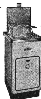
Modell Kg → Der zuverlässige Gasapparat Masse: 43,5×59,5×80 cm Ölbassin: Inhalt 9,5 l Gaskonsum 2500 l/h Fr. 1200.—
