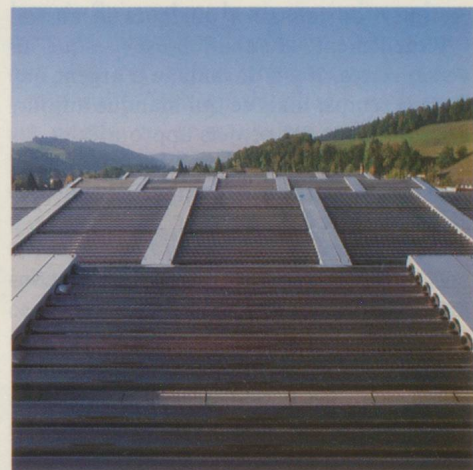
Une première mondiale: Une fabrique de pâtes suisse produit, au moyen d'une installation solaire placée sur le toit de l'usine, de la chaleur utilisable pour un processus industriel. (Photo: pd)
