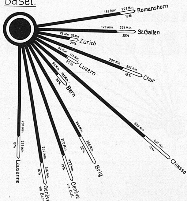
Kürzung der Reisedauer im Personenverkehr der SBB seit der Elektrifikation L'effet de l'électrification sur la durée des voyages en Suisse
