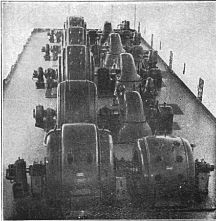
Maschinensaal d. Kraftwerkes Küblis d. A.-G. Bündner Kraftwerke, Leistung 47,000 PS
