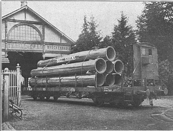
Elektrisch geschweisste Rohre zur Druckleitung Schlappin der Bündner Kraftwerke A.-G., Klosters — Erbaut 1927 — Länge der Rohrleitung: 2913 m; Durchm.: 900/800/750 mm
