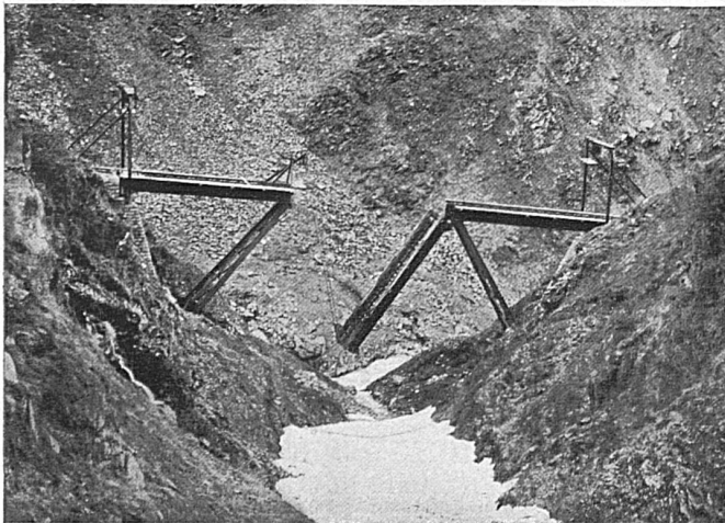
Steffenbachbrücke der Furka-Oberalp-Bahn - Diese Brücke wird jeden Winter wegen Lawinengefahr zusammengeklappt, auf die Widerlager zurückgelegt, und im Frühling wieder hochgezogen und zusammenmontiert
