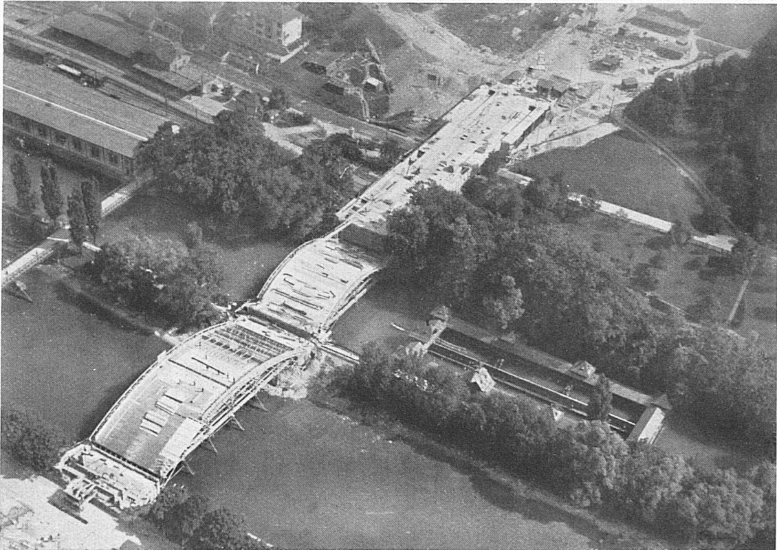
Kornhausbrücke Zürich
