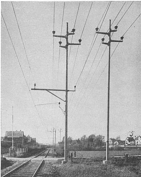
Sulzer-Masten bei Rapperswil
