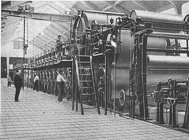
Rundsieb-Kartonmaschine für die Herstellung von Duplex- und Triplex-Kartons
