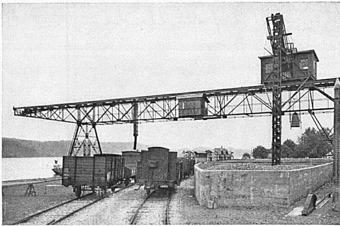
Verladebrücke der Seeverlad- und Kieshandels A.-G., Luzern Stützweite: 40 m; Gesamtlänge: 60,65 m
