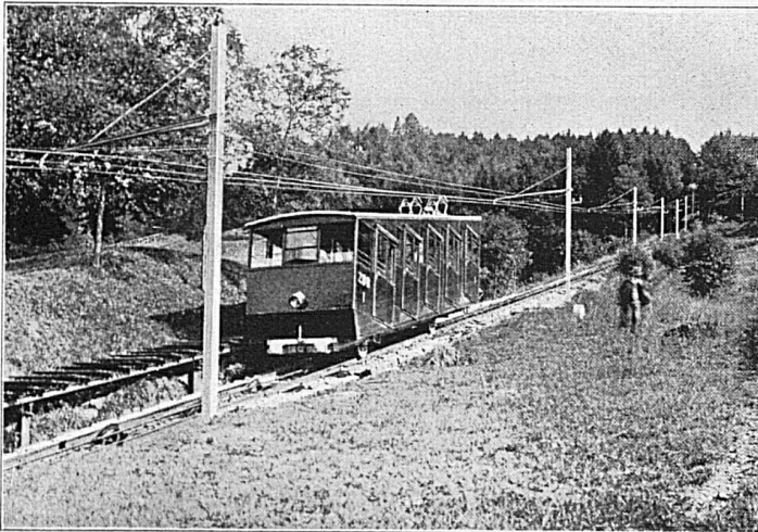
Drahtseilbahn auf den Zugerberg, kürzlich umgebaut für modernen Betrieb und grössere Leistungsfähigkeit
