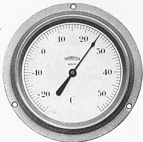
Le modèle applique, destiné à être encastré ou vissé sur cadre
