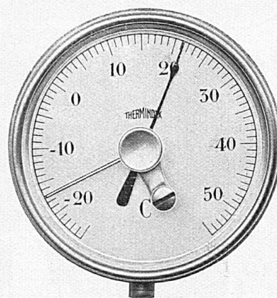
Le modèle mural, à contact électrique pour avertisseur
