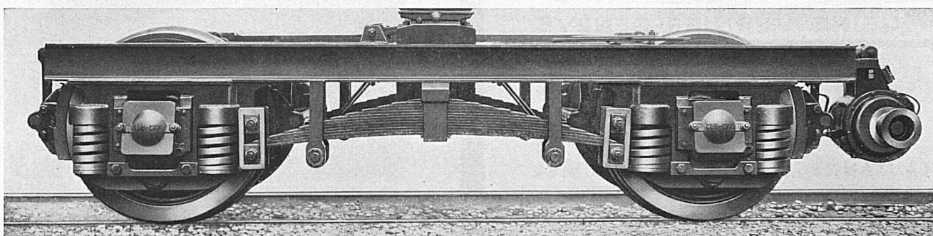
Neue geschweisste eiserne Bauart von Eisenbahnwagen der Schweizerischen Bundesbahnen
