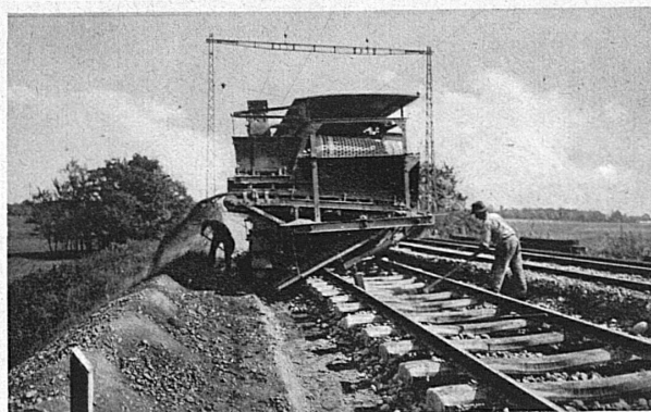
Machine à piocher, ameubler et désherber le ballast des voies de chemins de fer
