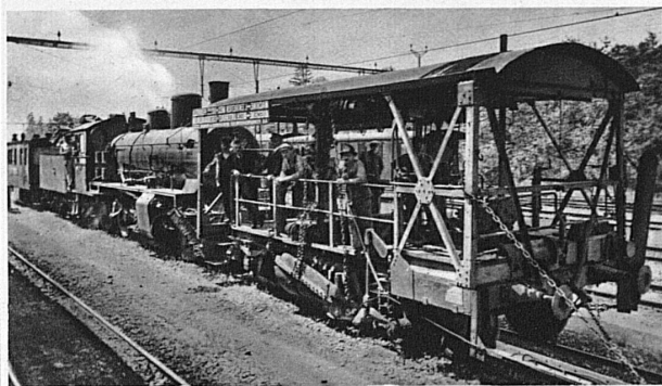
Machine à piocher, ameublir et désherber le ballast des voies de chemins de fer
