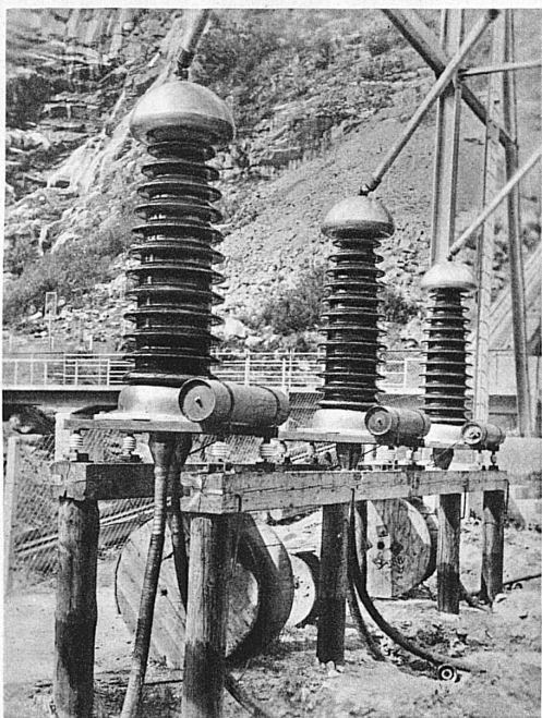
150 kV Ölkabelanlage in der Gotthardleitung Zentrale Piottino
