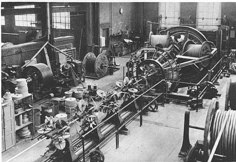
Blick in eine Fabrikations-Abteilung mit Hochspannungs-Verseilmaschine
