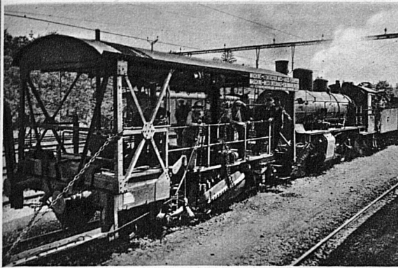
Machine à piocher, ameublir et désherber le ballast des voies de chemins de fer
