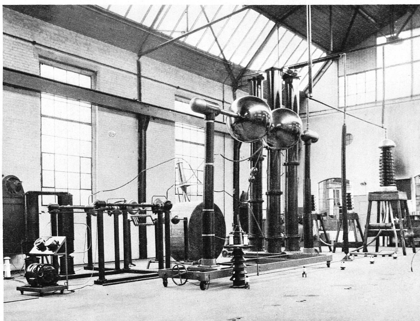
Stoßspannungsanlage für 1 Million Volt und 10000 Watt-sec. Leistung
