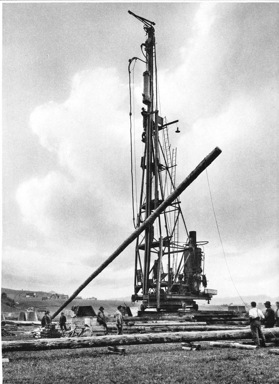
ETZELWERK: HOLZPFAHLFUNDATION DES VIADUKTES BEI WILLERZELL
