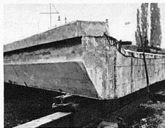
Die neue Brücke steht in Reserve, ein Ungeheuer im Gewicht von 400 Tonnen, auf eine Verschiebbahn aufmontiert, auf der sie in der kommenden Nacht an ihren Bestimmungsort gezogen werden soll
