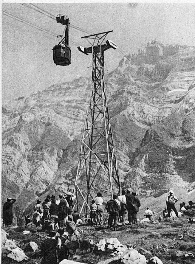
Stütze der Schwebebahn — Le téléphérique du Säntis au passage d'un pylone
