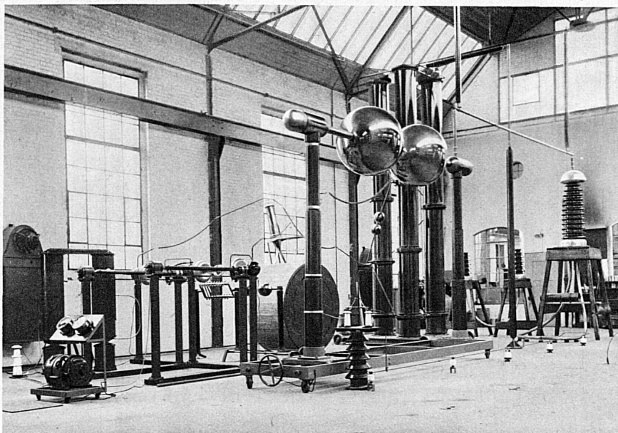
Stoss-Spannungsanlage für 1 Million Volt und 10000 Watt-sec. Leistung
