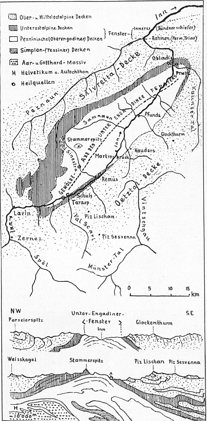
Das « Engadiner Fenster » mit den Heilquellen Tarasp, Schuls, Val Sinestra. Geostektonische Kartenskizze nach J. Cadisch, vereinfacht; zwei geologische Querprofile nach R. Staub, vereinfachte Ausschnitte.* Phot. und Profile: Leo Wehrli
