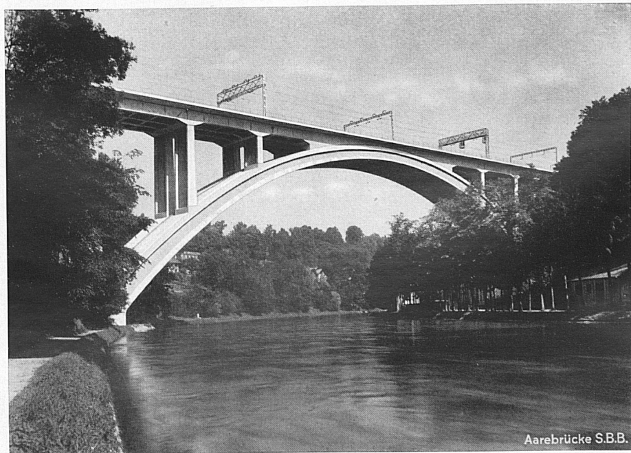
Aarebrücke und Viadukt SBB, aller Eisenbeton „pervibriert“
