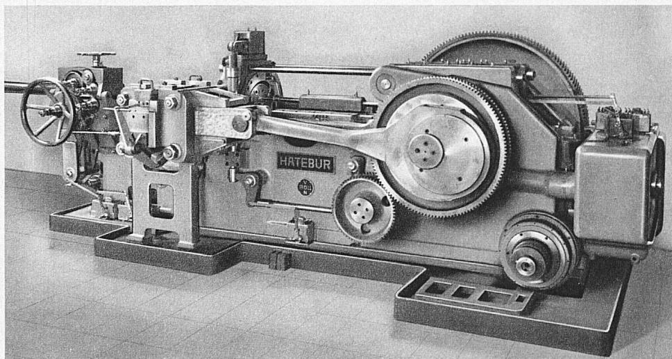
Autom. Warmpresse Type PWA-50
