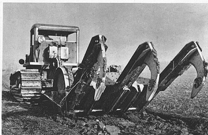
Tank - scarificateur. — Brevet E. G. T. 18 tonnes. — Capacité journalière de labourage 10.000 m 2 .
