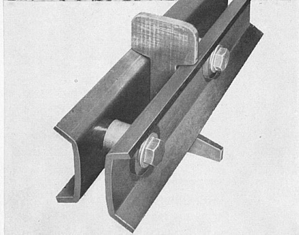
DELLITKÖRPER FÜR DIE ISOLATION VON EISENBAHNSCHIENEN
