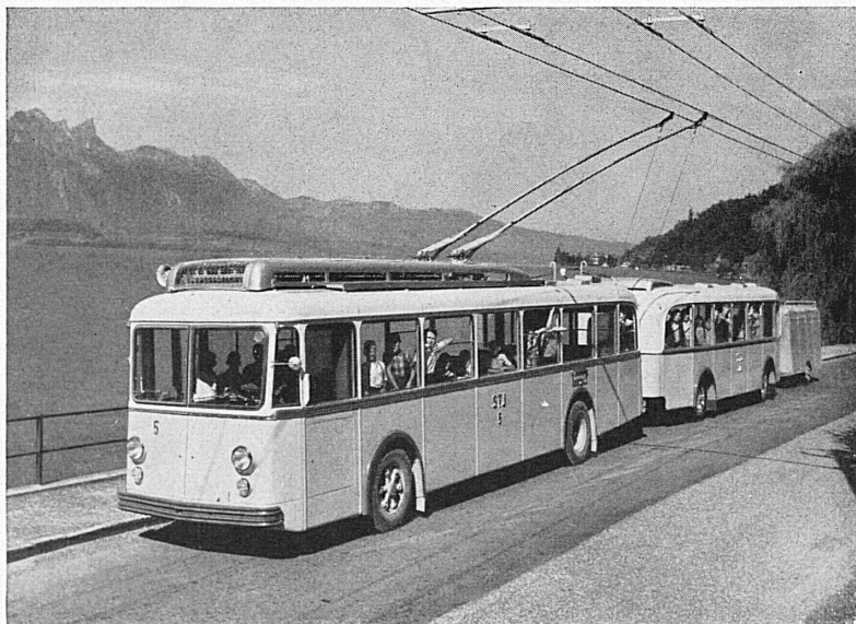
Rechtsufrige Thunerseebahn Un des 9 trolleybus équipés par Sécheron Tension 1000 V. Puissance: 160 ch. Vitesse maximum: 60 km/h.
