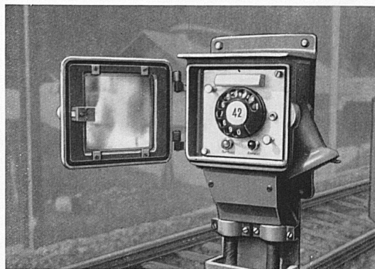
Gleismelder-Geberapparat
